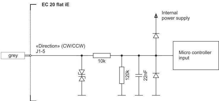
Figure 3-8 Input «Direction» – Internal circuitry
