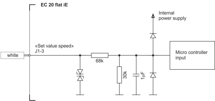
Figure 3-3 Input «Set value speed» – Internal circuitry
