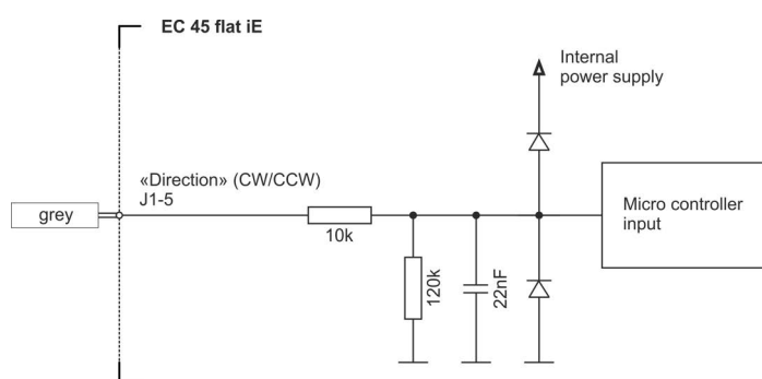
Figure 3-10 Input «Direction» – Internal circuitry
