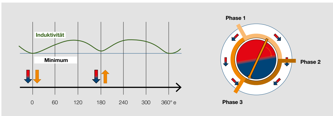
Abbildung 2: Schematische Darstellung der Anisotropie der Induktivität. Sie zeigt zwei fast identische Minima im Abstand von 180 elektrischen Grad.
