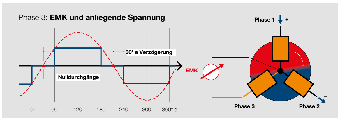
Abbildung 1: Schematische Darstellung der sensorlosen Kommutierung der EMK-Methode mit Nulldurchgang, hier am Beispiel der Phase 3 gezeigt.
